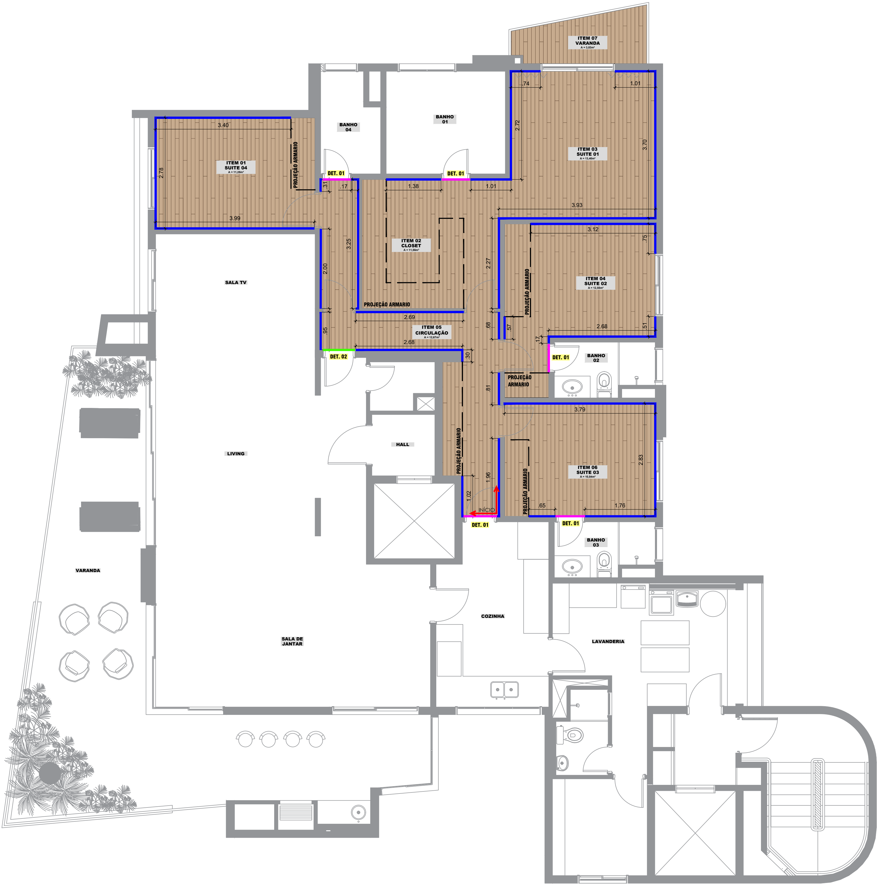
PLANTA DE PAGINAÇÃO DE PISO 1:50
