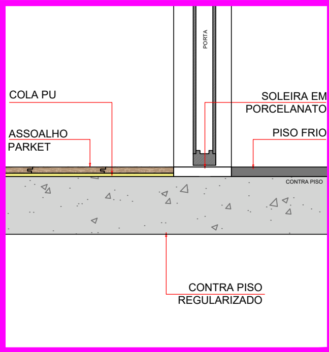
DET. 01 - TRANSIÇÃO DE PISO 1:10
