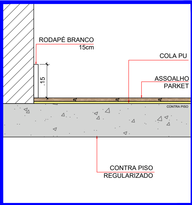
DET. RODAPÉ 1:10
